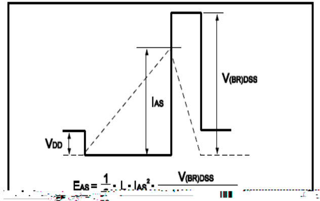
Fig.14 Avalanati Waveform
